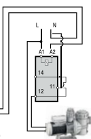
FILTRAČNÍ ČERPADLO Kontrola filtrace 9 a 10
